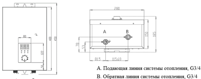
Рис. 9. Присоединительные размеры
