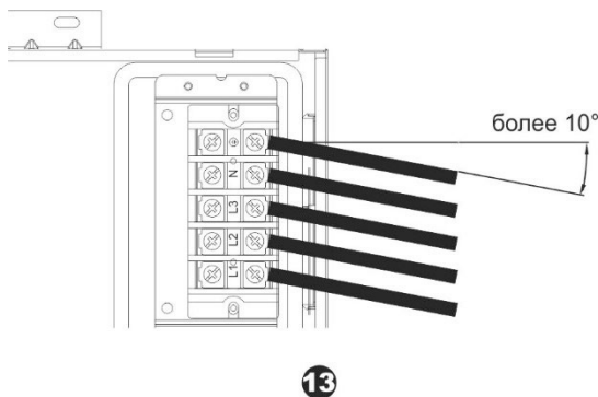
Рис. 14. Расположение сетевого кабеля
