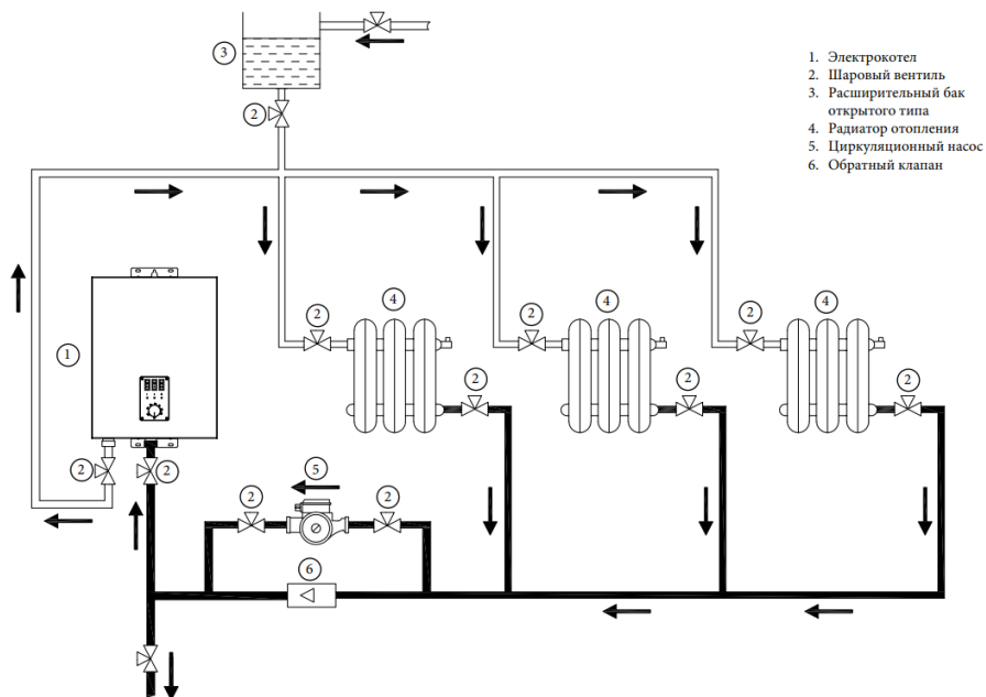
Рис. 6. Схема подключения в систему с естественной циркуляцией
