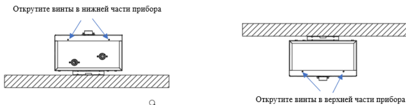
Рис. 10. Демонтаж лицевой панели
