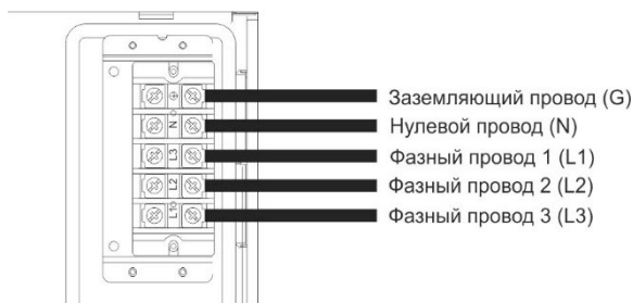
Рис 13. Трехфазное подключение прибора
