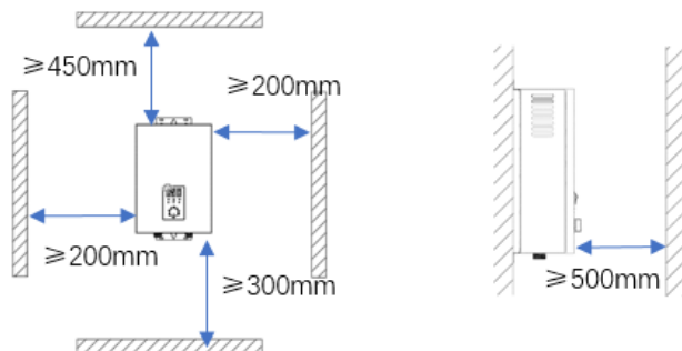
Рис. 7. Минимальные расстояния от электрического котла до поверхностей.
