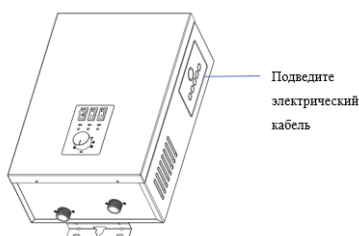
Рис. 11. Расположение панели вывода электрического кабеля
