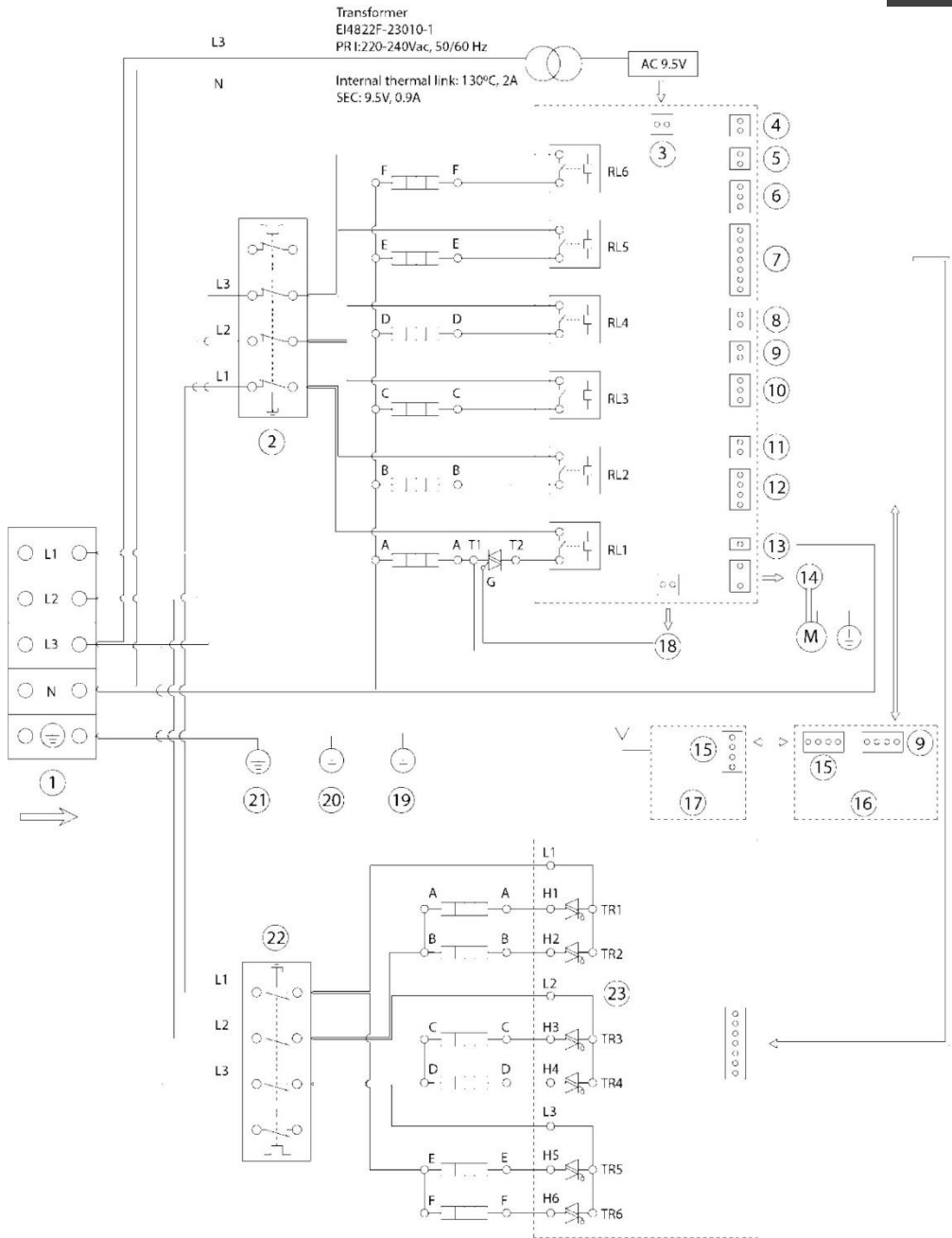
Рис.11. Электрическая схема
