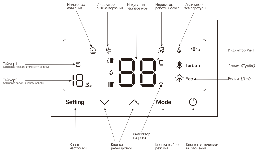
Рис. 3. Панель управления
