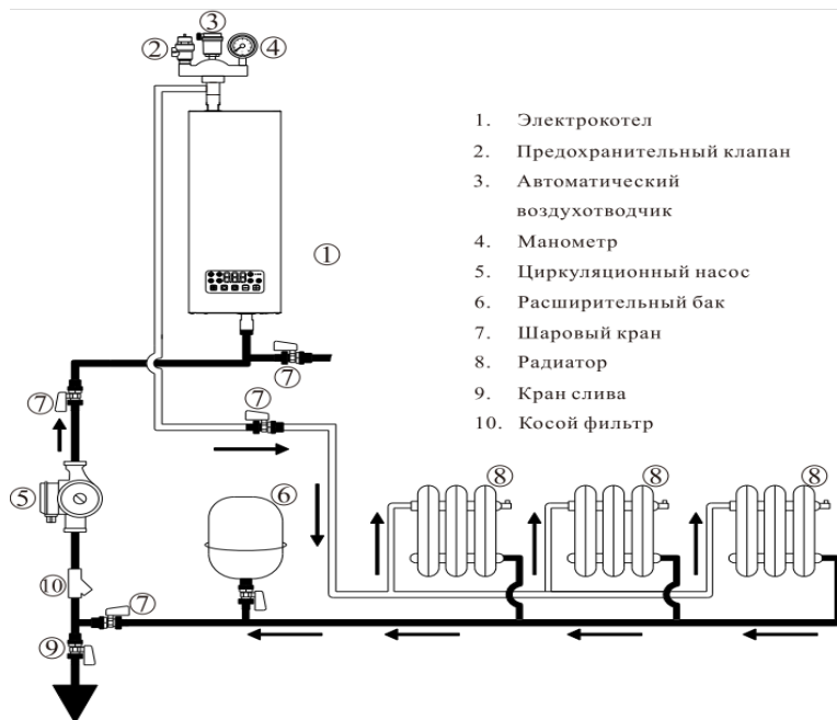
Рис. 4. Схема подключения в систему с радиаторным отоплением.
