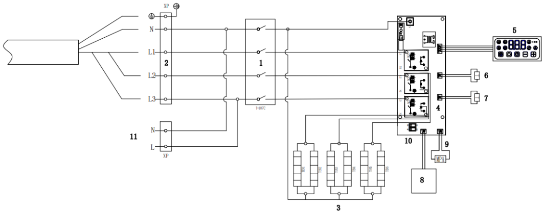
Рис. 14. Электрическая схема THERMEX Maia 6
