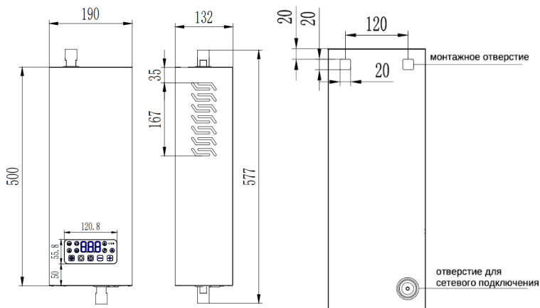
Рис. 9. Монтажные размеры
