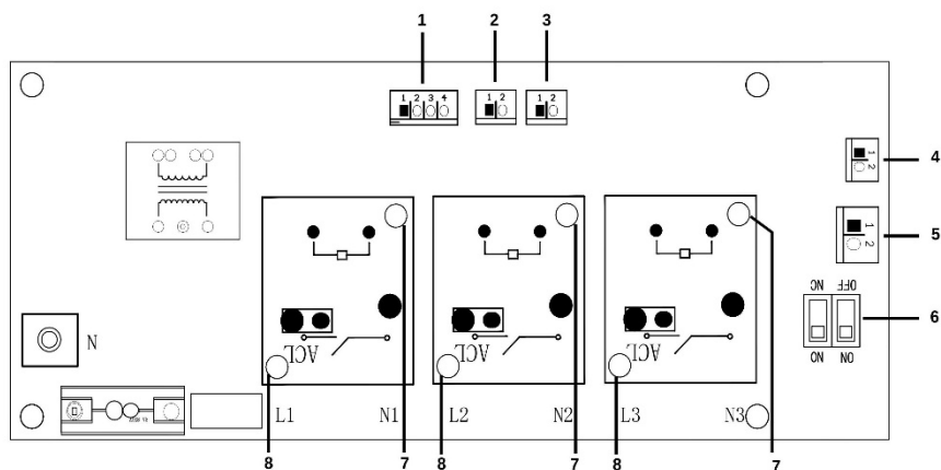
Рис. 15. Электрическая схема основной платы управления
