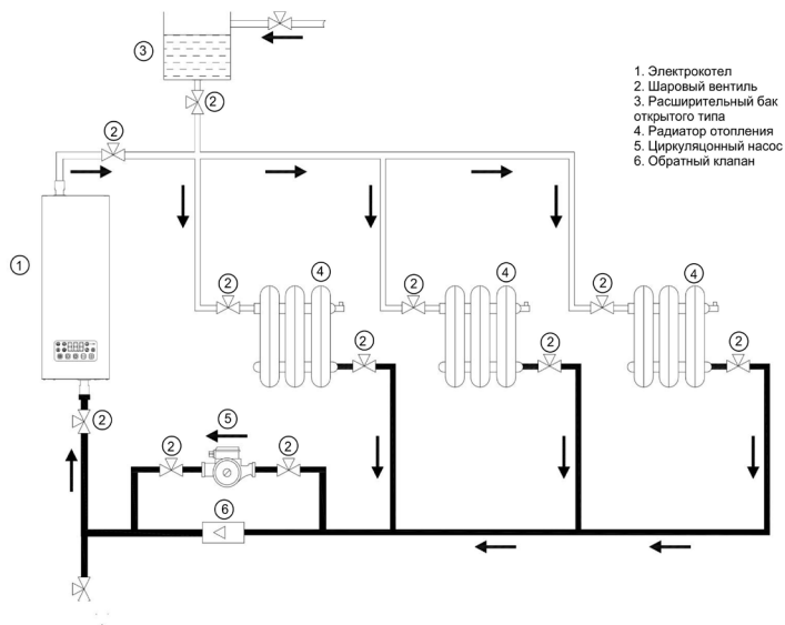
Рис. 7 Схема подключения в систему с естественной циркуляцией.
