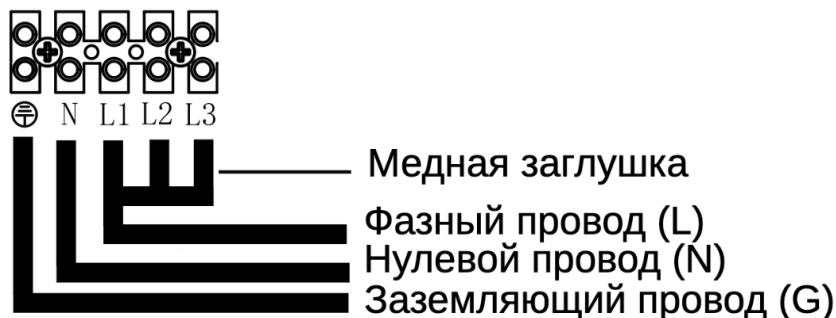
Рис 12. Однофазное подключение прибора
