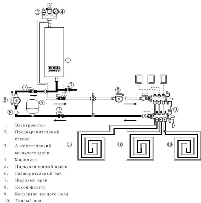
Рис. 6. Схема подключения в систему отопления радиаторы + теплый пол.
