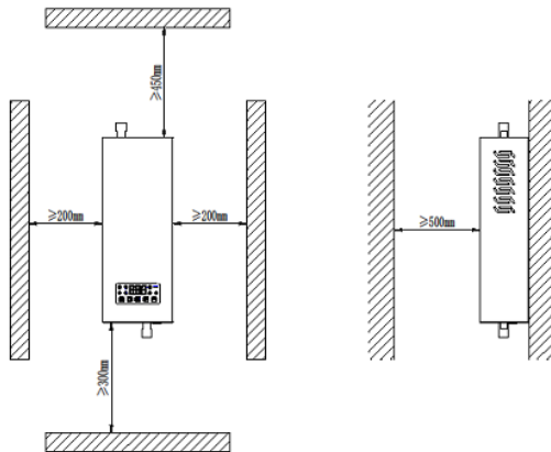
Рис. 8. Минимальные расстояния от электрического котла до поверхностей.
