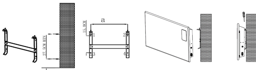
Рис.2 Установка на стену
