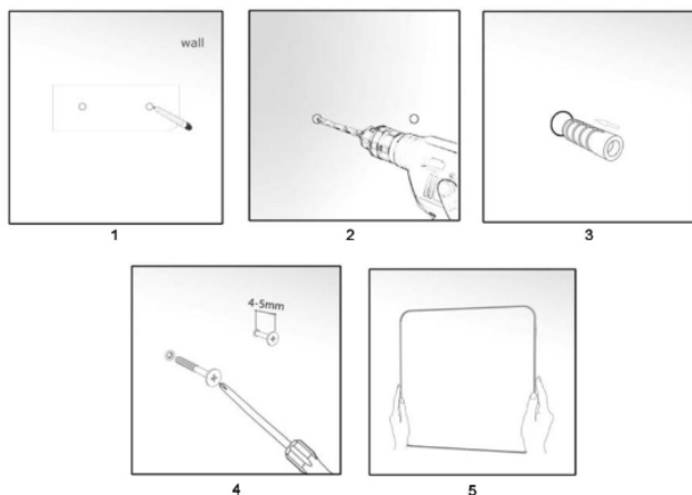
Рис. 3. Монтаж устройства
