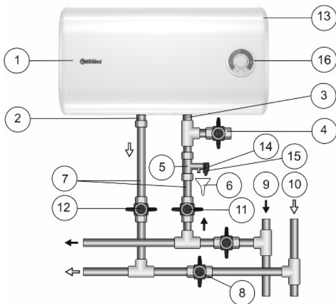
Рисунок 1-2. Схема подключения ЭВН к водопроводу в вертикальном и горизонтальном положениях
