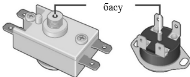
3-сурет. Термоажыратқыш түймешігінің ықтимал орналасу сұлбасы
